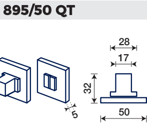
NOTTOLINO WC CON ROSETTA BASSA QUADRATA THUMBTURN WITH THIN SQUARE ROSE
