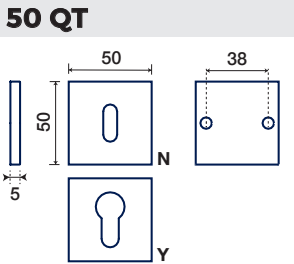
BOCCHETTA QUADRATA BASSA THIN SQUARE ESCUTCHEON
