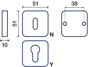
BOCCHETTA QUADRATA CON ANGOLI RAGGIATI RADIUS SQUARE ESCUTCHEON
