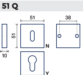
BOCCHETTA QUADRATA SQUARE ESCUTCHEON
