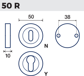
BOCCHETTA Ø 50 mm ESCUTCHEON Ø 50 mm
